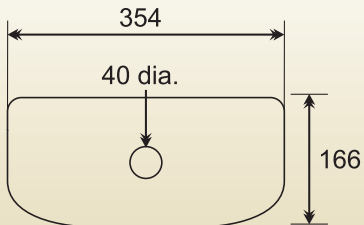
Top Elevation
